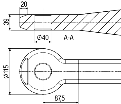
Anneau suisse 40 mm (p.e. ROCKINGER Typ ROE57229)
