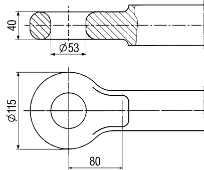
Anneau 40 mm DIN 74054 et EC classe S
