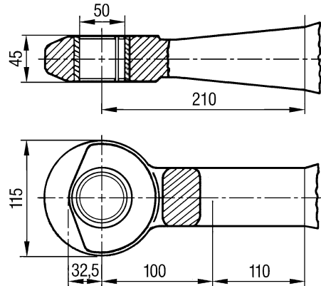
Anneau 50 mm DIN 74053 et EC classe D
